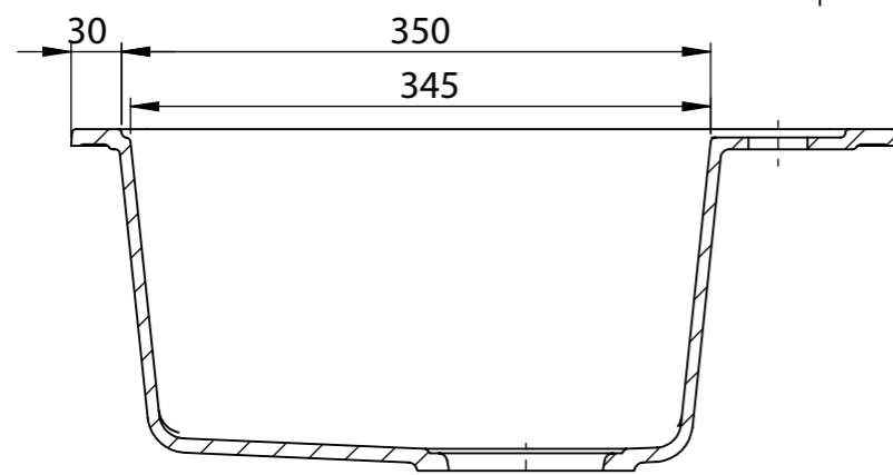
B-B
